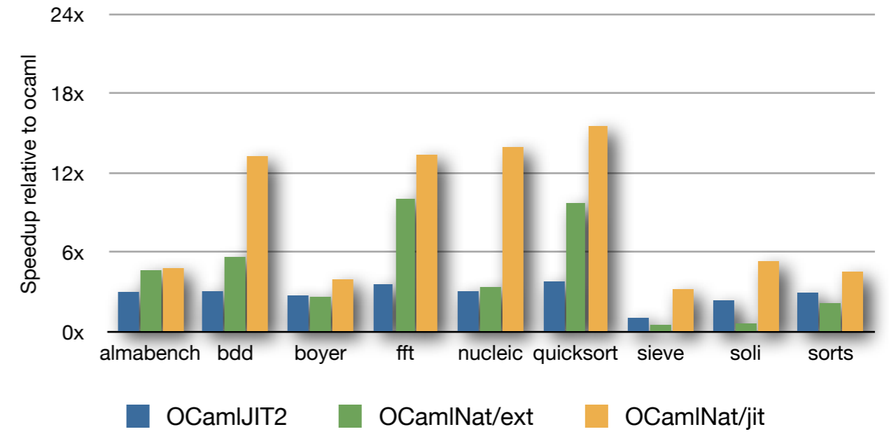
Intel Xeon, CentOS 5.6 (amd64)
